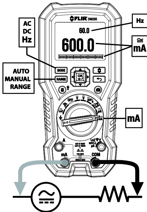
Fig. 9-10 mA Stroommetingen
