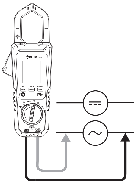
Figuur 5.1 Spanningsmetingen
